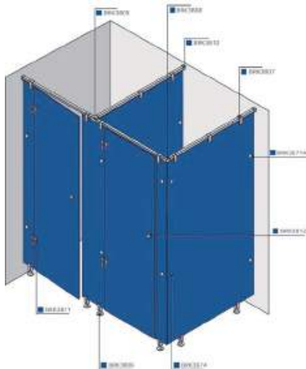
Diagrama herrajes para baño cuadrado
